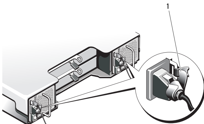
图 16-12. 固定电源电缆
